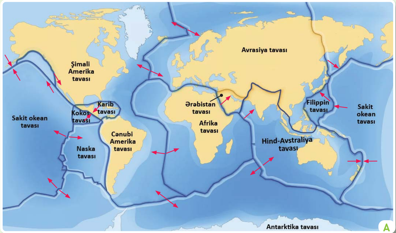
Litosfer tavaları
