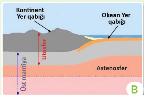
Litosfer təbəqəsi
