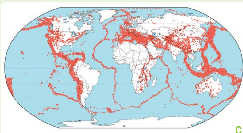
Zəlzələ ocaqları
