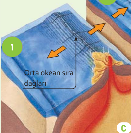
Litosfer təbəqəsi
