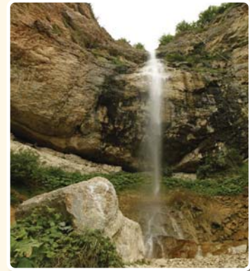
Afurca şlaləsi
