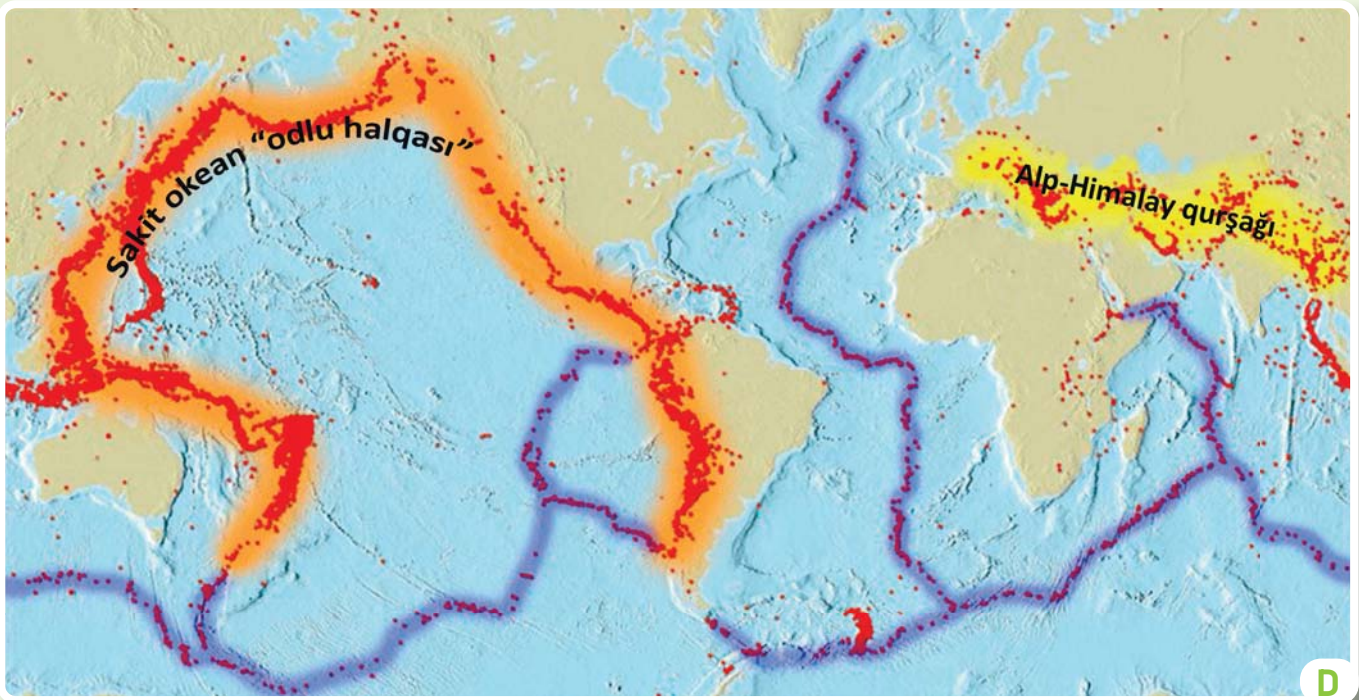
Seysmik qurşaqlar
