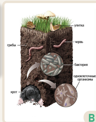
Органический состав почвы
