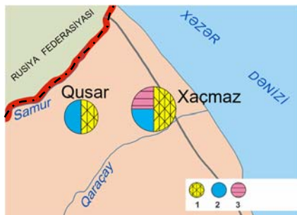
Kartodiaqram. “Sənaye sahələri”
