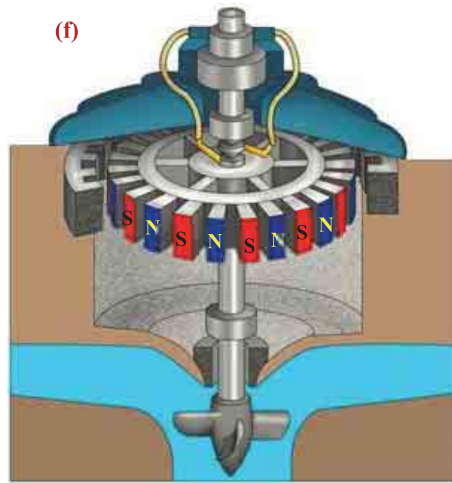
Hidrogenatorun sxemi
