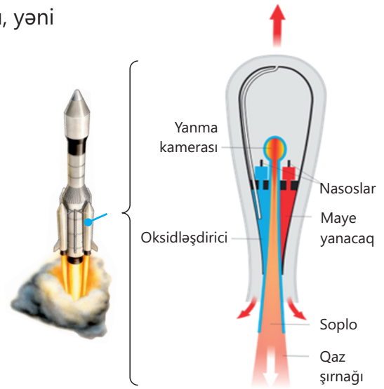
Şəkil 6.13. Raket mühərrikinin iş prinsipinin sxemi
