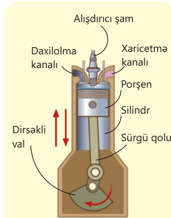
Şəkil 6.9. Daxiliyanma mühərrikinin silindri (quruluşu)
