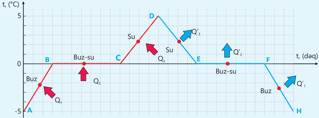
Şəkil 6.2. Buzun ərimə və suyun donma (bərkimə) prosesinin temperatur-zaman qrafiki.
