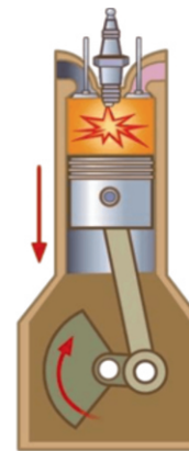
Şəkil 6.10. Dördtaktlı karbürətorlu mühərrikin iş prinsipi
