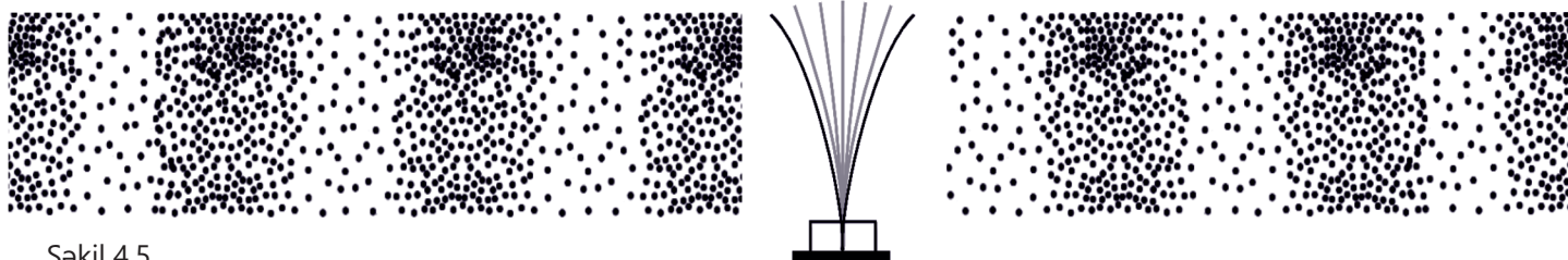
Şəkil 4.5. Səs havada uzununa dalğadır
