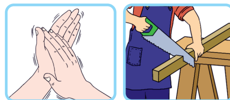
Şəkil 5.7. Daxili enerjinin mexaniki işgörmə ilə artması
