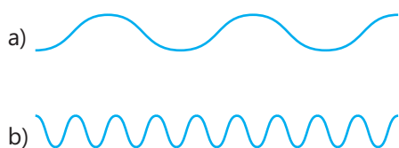
Şəkil 4.9. Müxtəlif rəqş tezlikli kamertonlarda müxtəlif tonlu səslər alınır.
