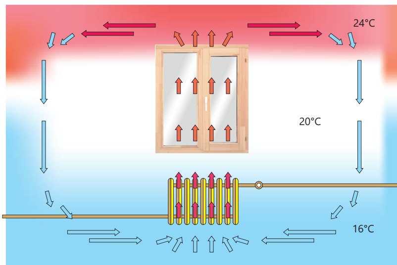
Şəkil 5.10. Qazlarda konveksiya
