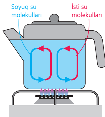
Şəkil 5.9. Mayədə konveksiya
