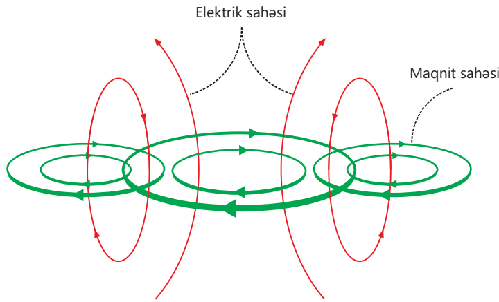
4.17. Elektromaqnit dalğası
