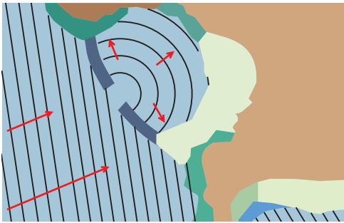
Su səthində yayılan dalğaların difraksiyası
