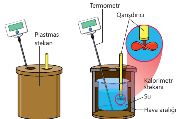
Şəkil 6.1. Laboratoriya kalorimetri
