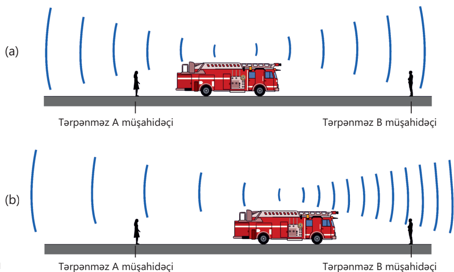
Şəkil 4.10. Dopler effektinin təzahürü
