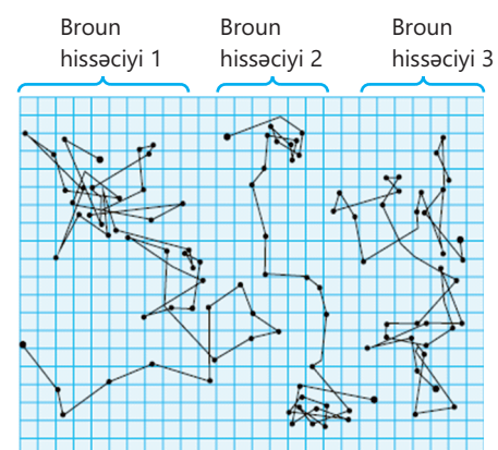
Şəkil 5.1. Broun hissəciklərinin hərəkət trayektoriyası
