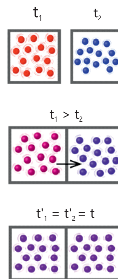
Şəkil 5.5. Cisimlər arasında istilik tarazlığının yaranması
