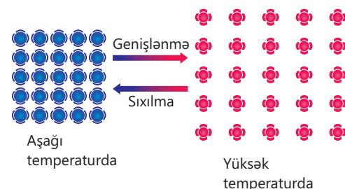
Şəkil 5.4. Bərk cismin istidən genişlənməsi, soyuqdan sıxılması
