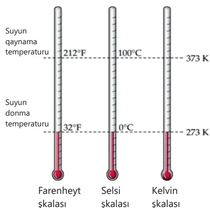
Şəkil 5.6. Temperatur şkalaları
