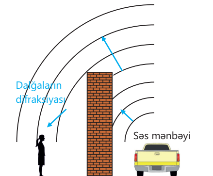
Səsin difraksiyası
