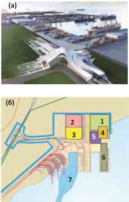
Общий вид проекта (а) и схема (б)
