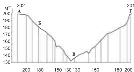
Профиль местности на основе горизонталей по линии А – Г на топографической карте
