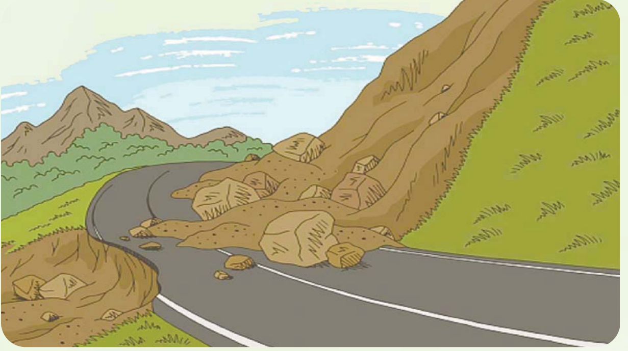
Torpaq sürüşməsi
