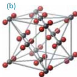
Karbon-dioksid
