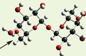
Строение сахара
