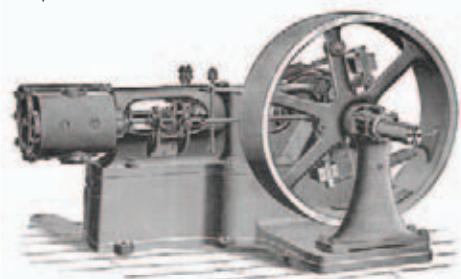
Паровой двигатель
